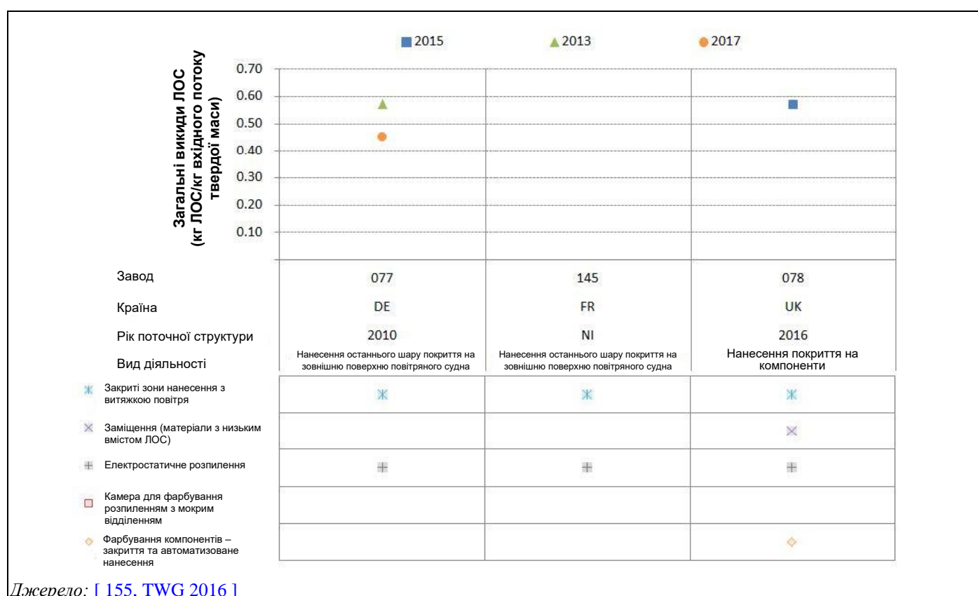
Рисунок 5.4: Загальні викиди ЛОС, виражені в кг ЛОС на кг вхідного потоку твердої маси
