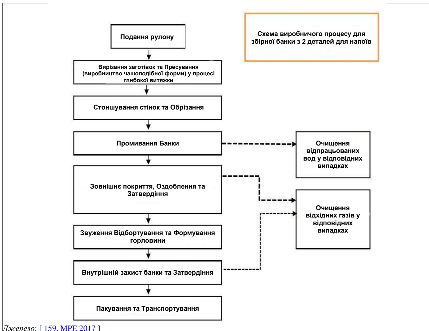
Рисунок 10.1: Процес виробництва банок для напоїв
