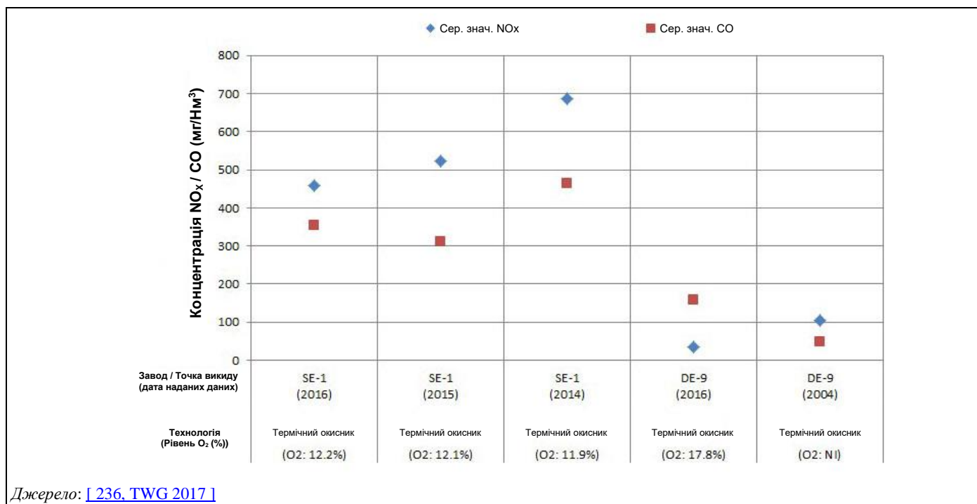
Рисунок 15.17: Повідомлені викиди NO x та CO у відпрацьованих газах від заводів із використанням креозоту
