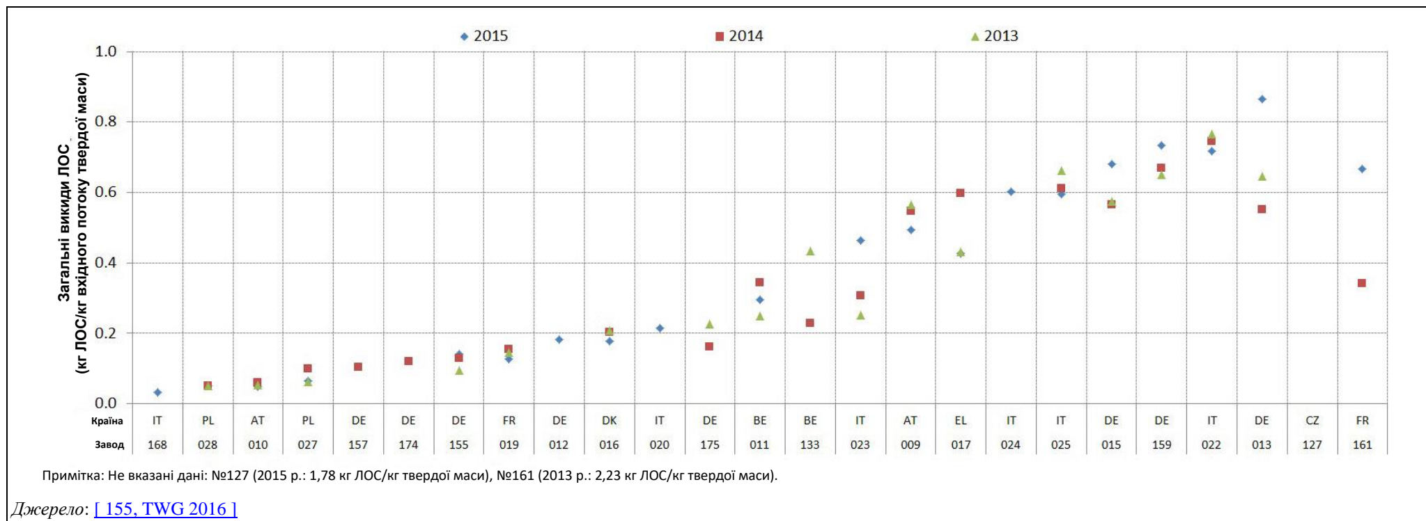
Рисунок 12.3: Загальні викиди ЛОС, виражені в кг ЛОС на кг вхідного потоку твердої маси за період 2013–2015 рр.
