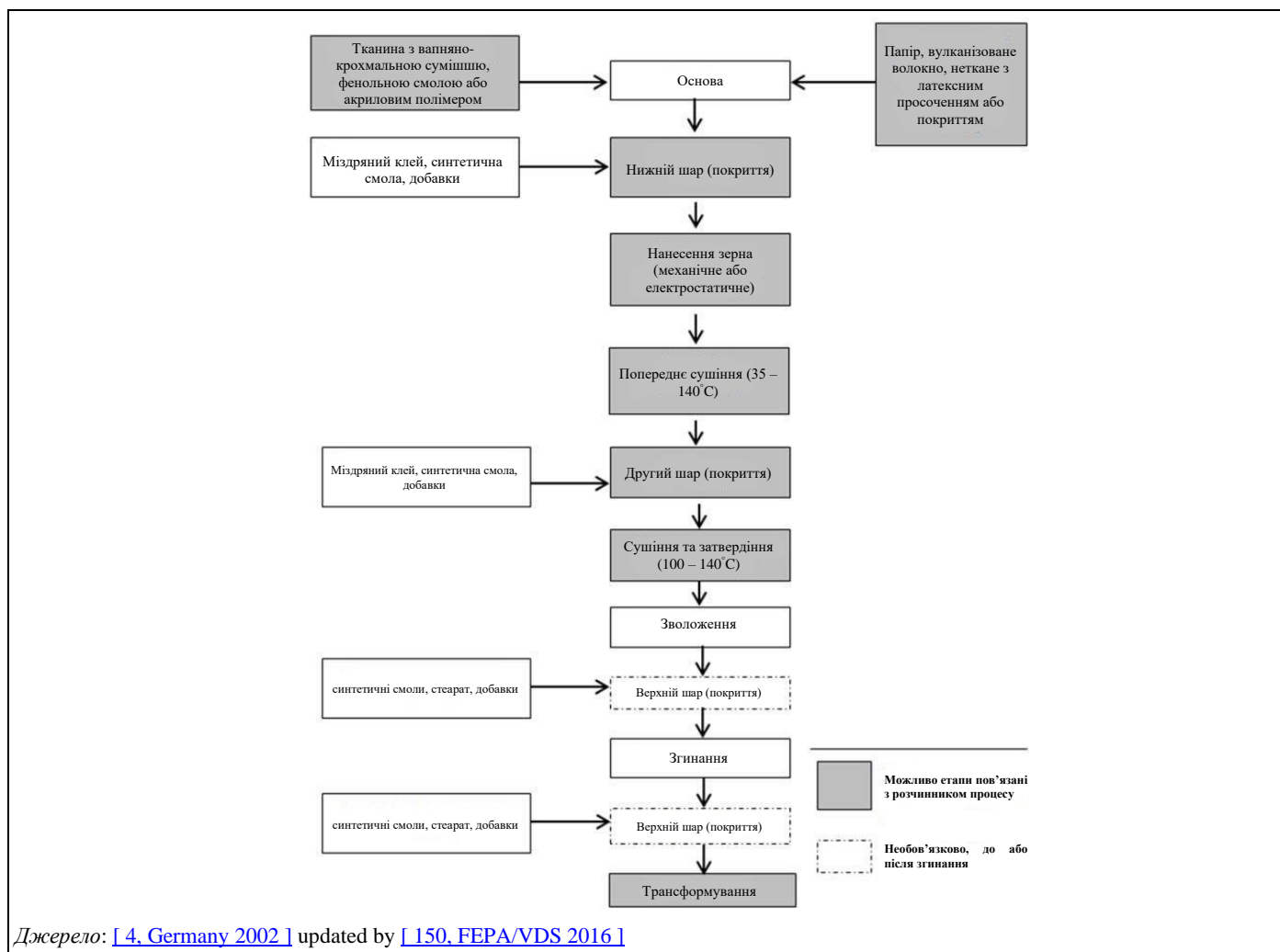
Рисунок 16.3: Схема процесу для абразивів із покриттям
