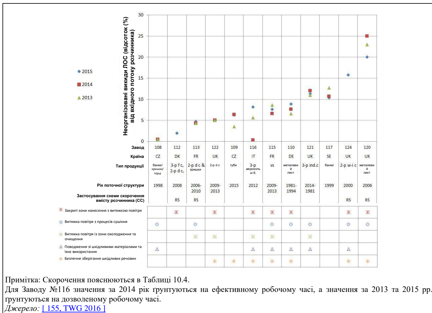
Рисунок 10.13: Неорганізовані викиди ЛОС, виражені як відсоток від вхідних потоків розчинника за період 2013–2015 рр.
