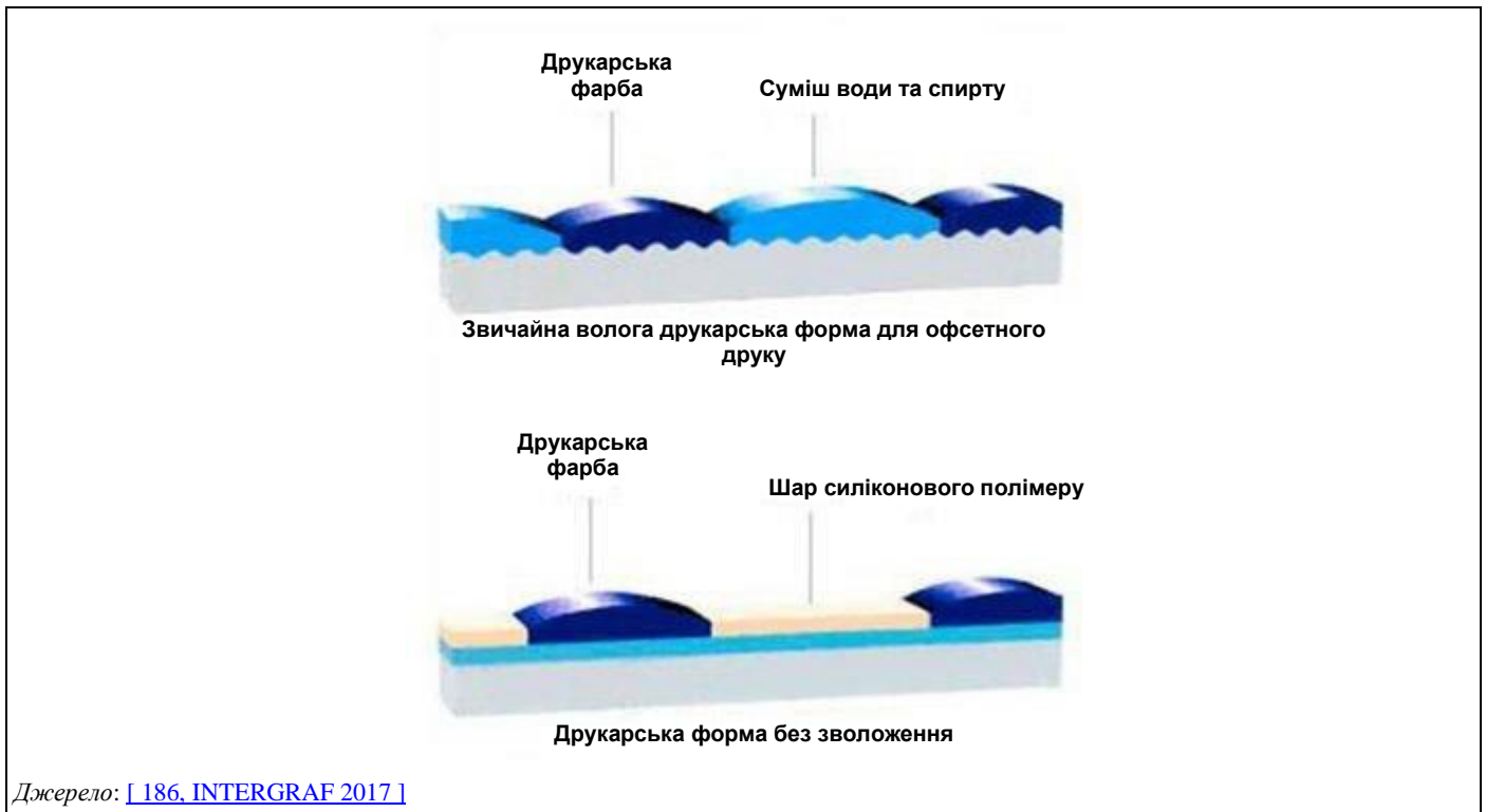
Рисунок 11.11: Звичайна друкарська форма для офсетного друку зі зволоженням та друкарська форма без зволоження
