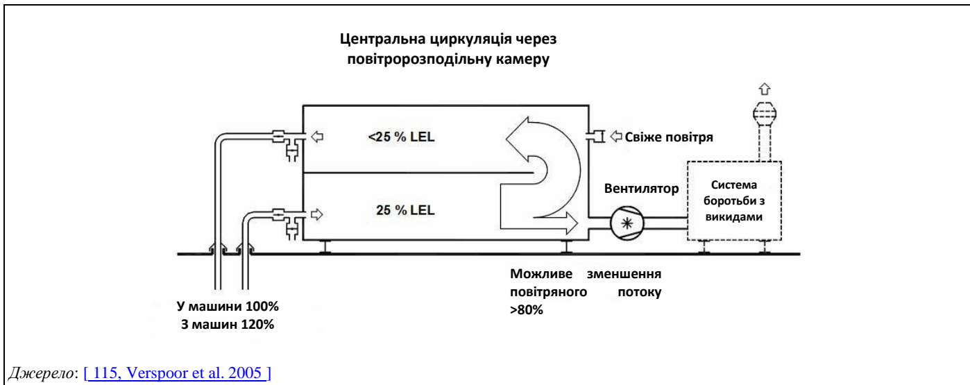
Рисунок 17.22: Повітророзподільна камера
