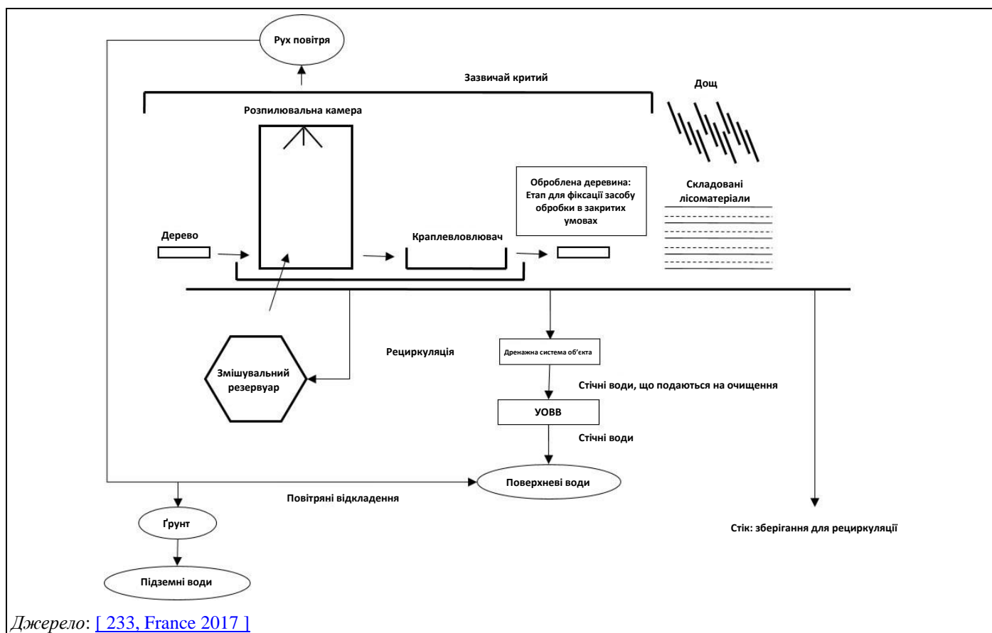
Рисунок 15.6: Схема процесу розпилення / розпилювального тунелю
