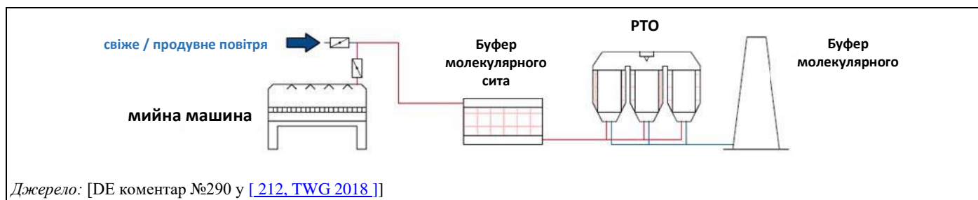
Рисунок 17.19: Схема системи очищення вихлопних газів із буфером молекулярного сита
