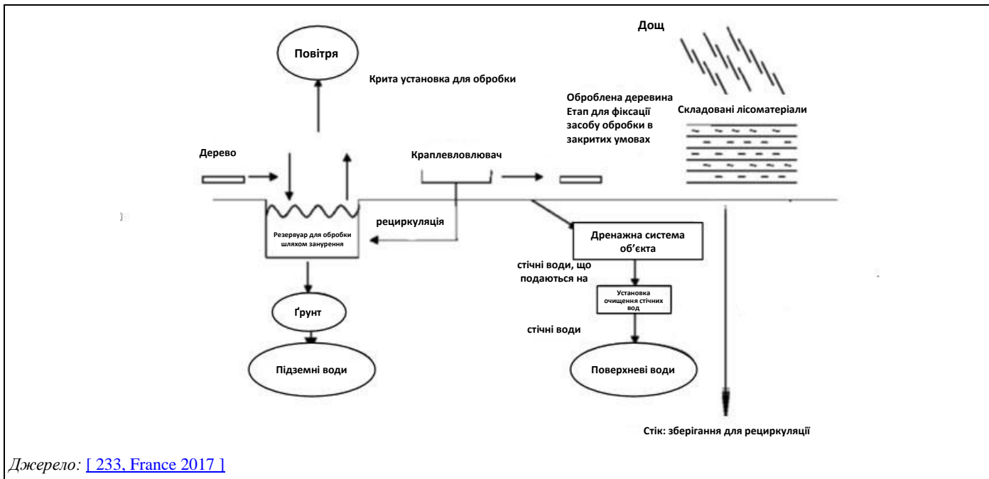
Рисунок 15.4: Схема процесу короткочасного занурення (короткострокове занурення/занурення на певний час)
