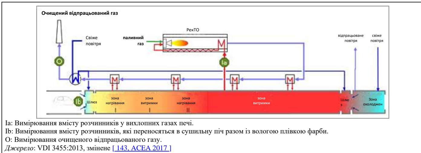
Рисунок 21.5: Точки вимірювання для визначення ефективності боротьби з викидами на установках з очищення відхідних газів у комбінації очищення відхідних газів сушильної печі
