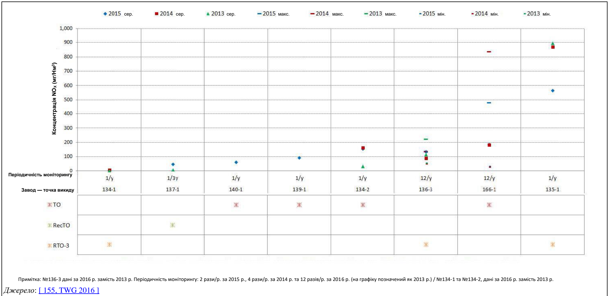
Рисунок 8.7: Викиди NOx у відпрацьованих газах за період 2013–2015 рр. (періодичний моніторинг)
