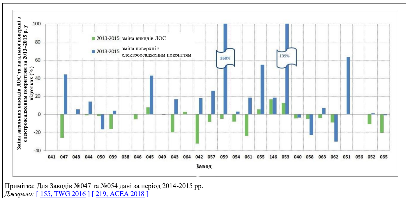
Рисунок 2.21: Зміна загальних викидів ЛОС (г/м 2 ) та загальної поверхні з покриттям, нанесеним електроосадженням за 2013–2015 р. у відсотках
