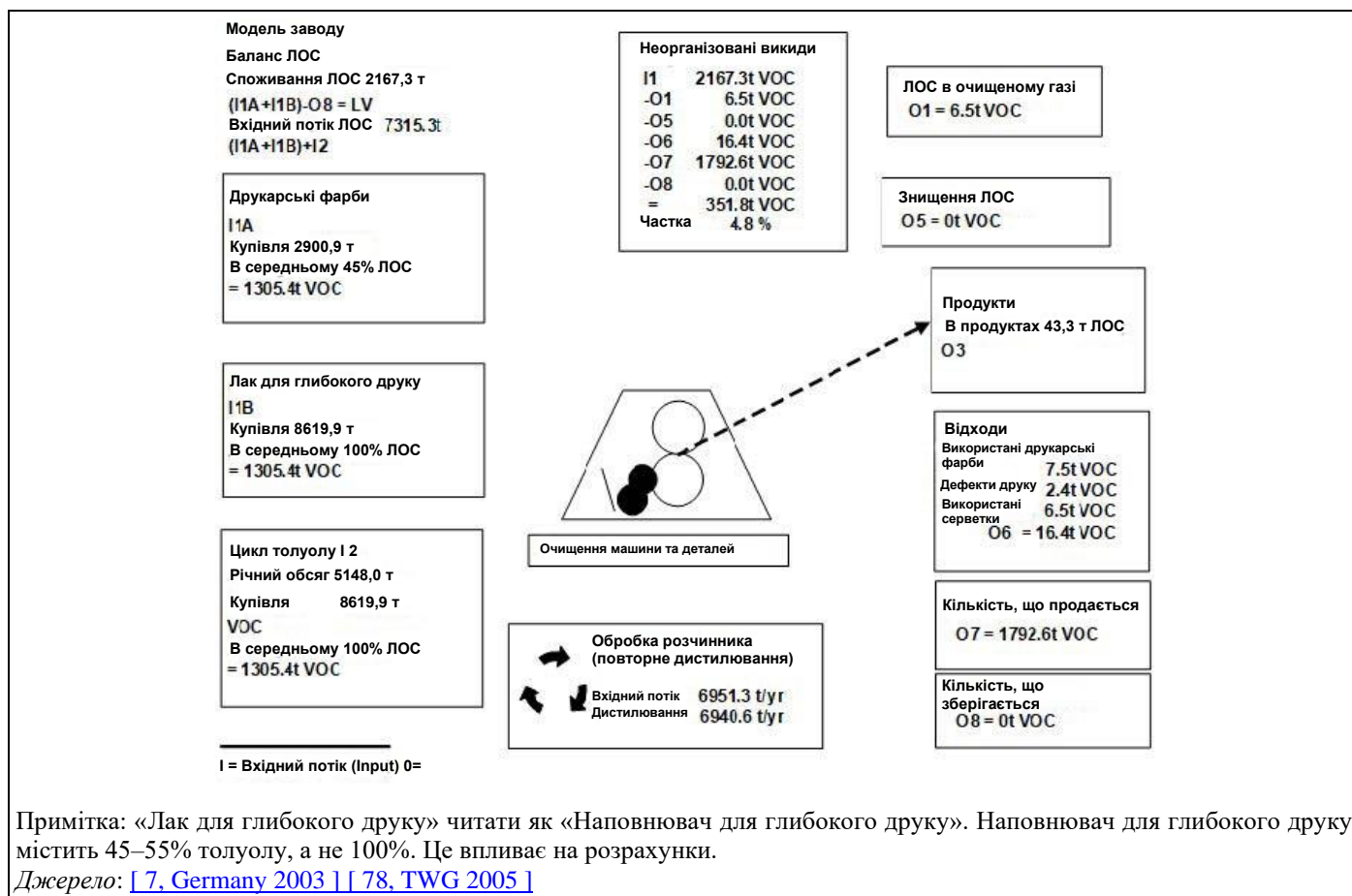
Рисунок 13.2: Баланс ЛОС віртуального заводу публікаційного ротогравюрного друку
