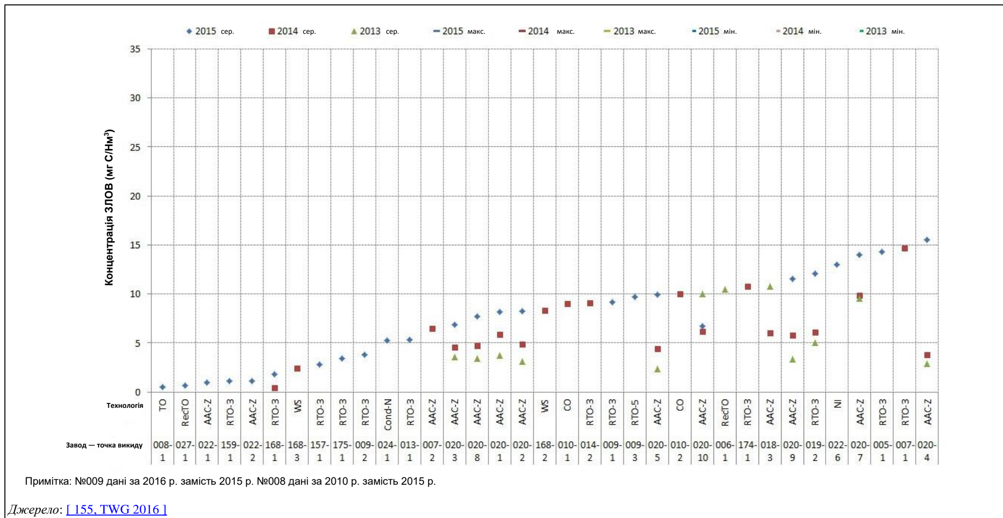
Рисунок 12.5: Викиди ЗЛОВ у відпрацьованих газах (періодичний моніторинг) за період 2013–2015 рр. (1/2)
