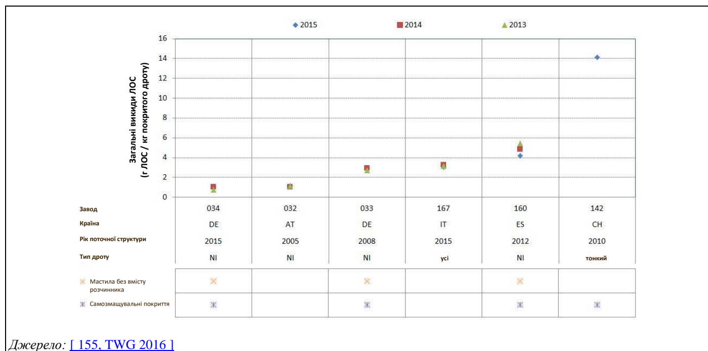
Рисунок 9.2: Загальні викиди ЛОС, виражені у г ЛОС на кг покритого дроту за період 2013–2015 рр.
