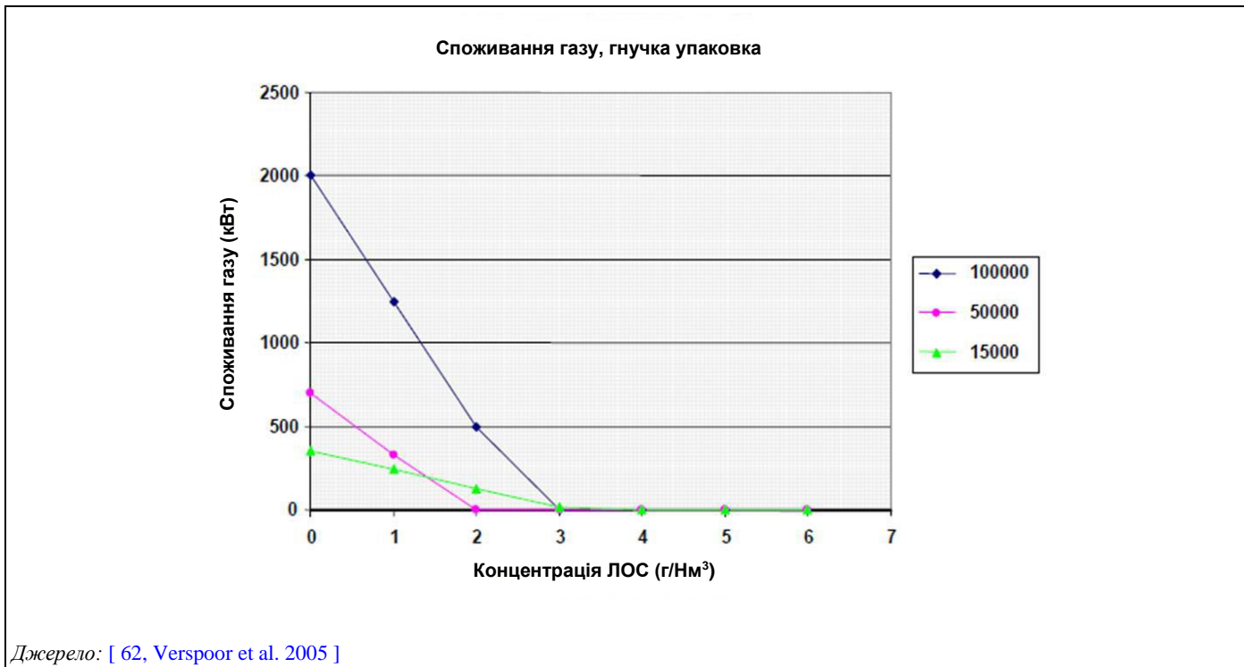
Рисунок 17.16: Приклад споживання газу нижче автотермічної точки для заводу з флексографічного друку та публікаційного ротогравюрного друку для трьох сценаріїв витрати
