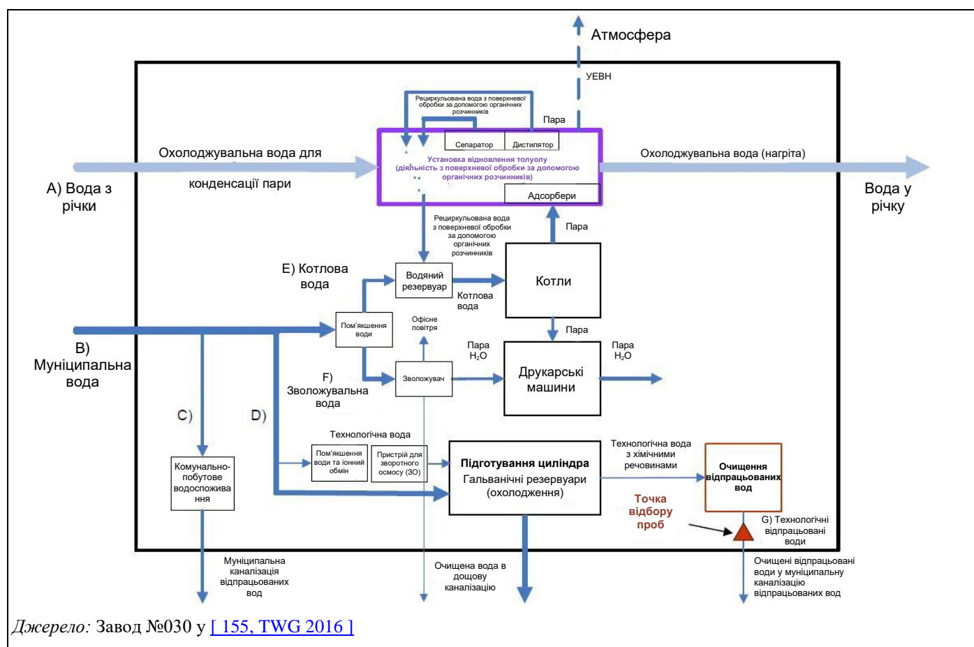
Рисунок 13.4: Схема використання води на установці з публікаційного ротографічного друку
