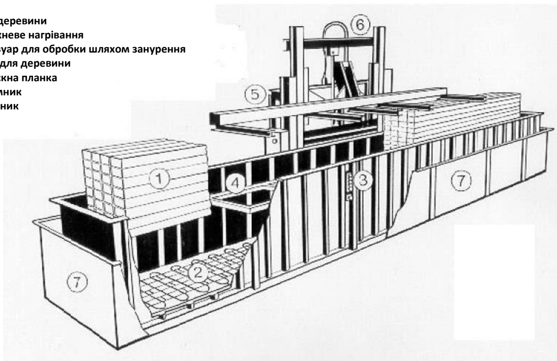
Рисунок 15.8: Схема просочення у ванні
