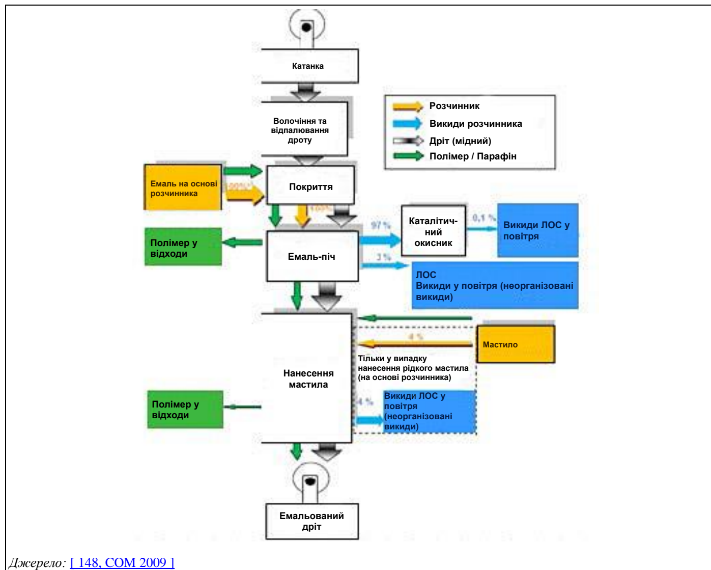
Рисунок 9.1: Типовий виробничий процес та схема виробництва обмоткового дроту
