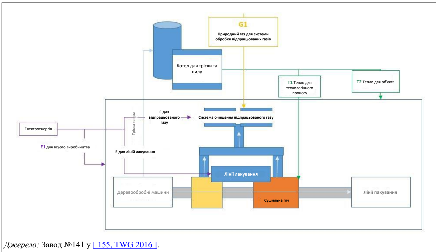
Рисунок 14.2: Схема вхідних потоків енергії
