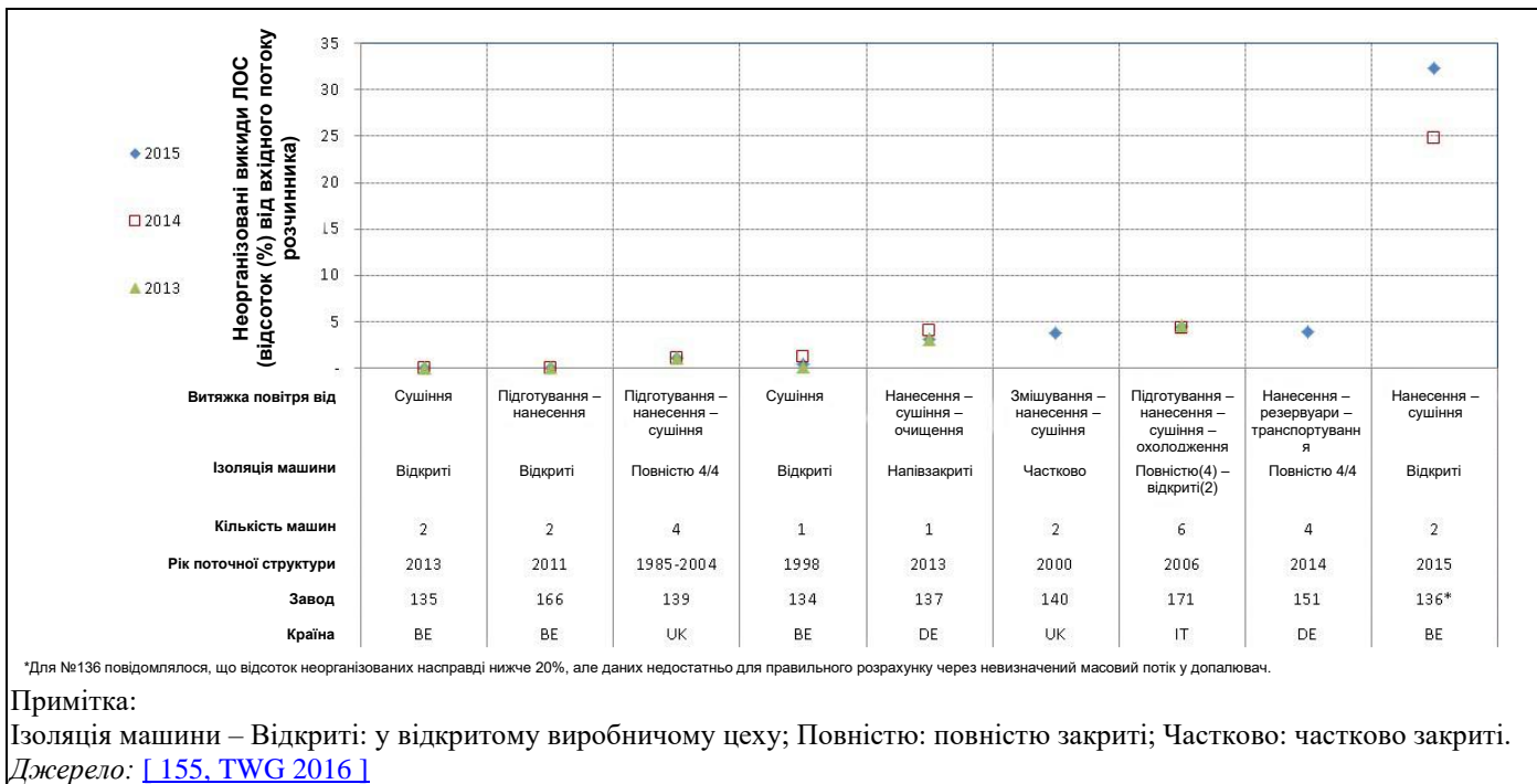
Рисунок 8.3: Неорганізовані викиди ЛОС, виражені як відсоток від вхідних потоків розчинника за період 2013–2015 рр.
