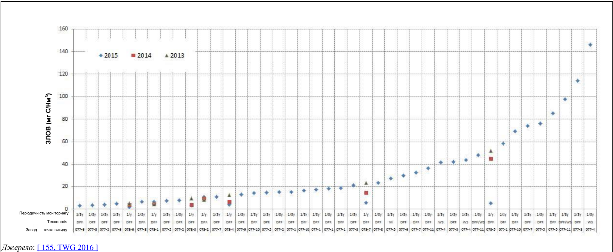
Рисунок 5.6: Викиди ЗЛОВ у відпрацьованих газах (періодичний моніторинг) – Середні значення за період 2013–2015 рр.
