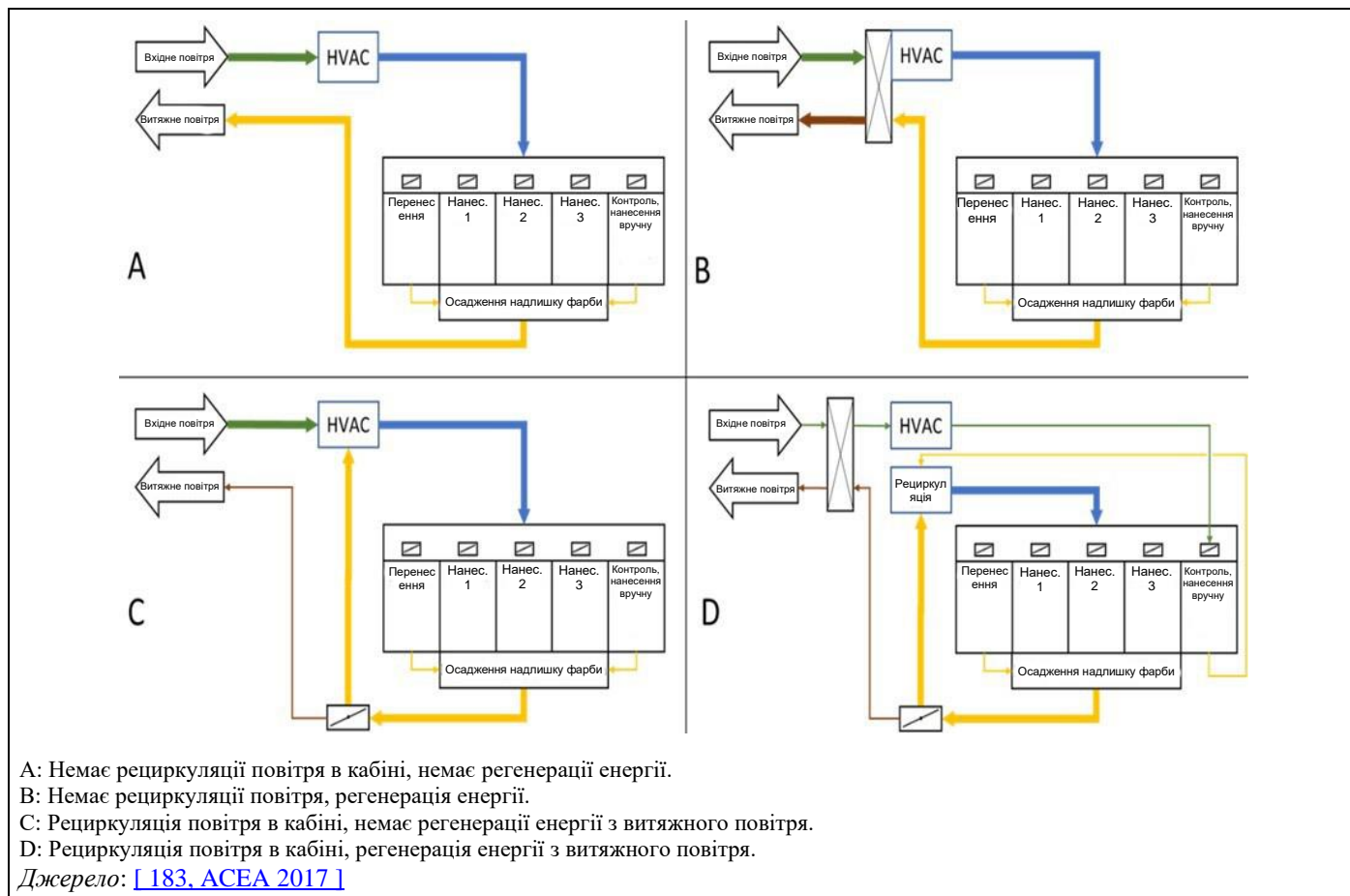
Рисунок 2.44: Різні варіанти спрямування повітря та регенерації енергії
