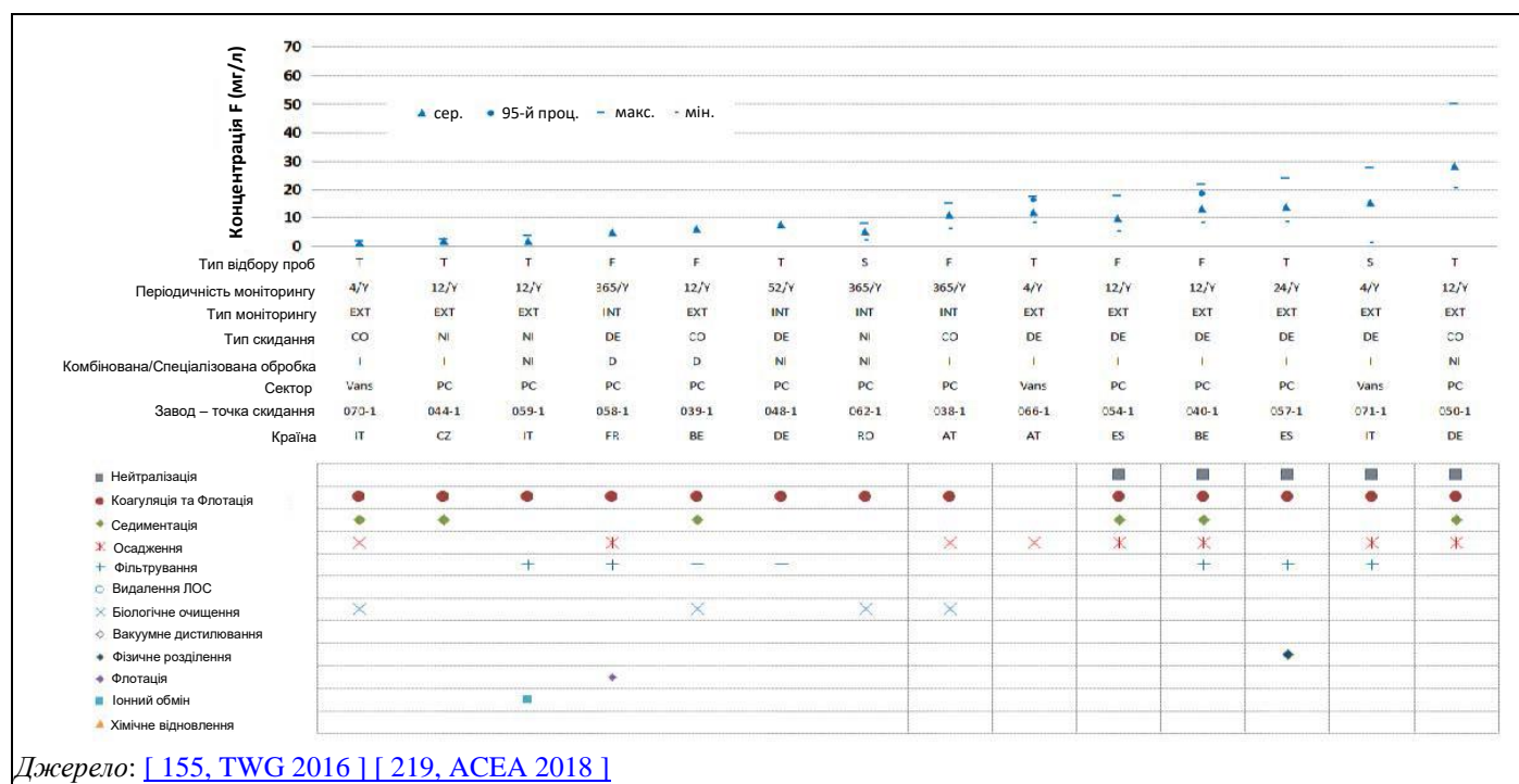
Рисунок 2.36: Значення концентрації фторидів для прямого та непрямого скидання стічних вод заводів із нанесення покриття на транспортні засоби (дані за 2015 р.)
