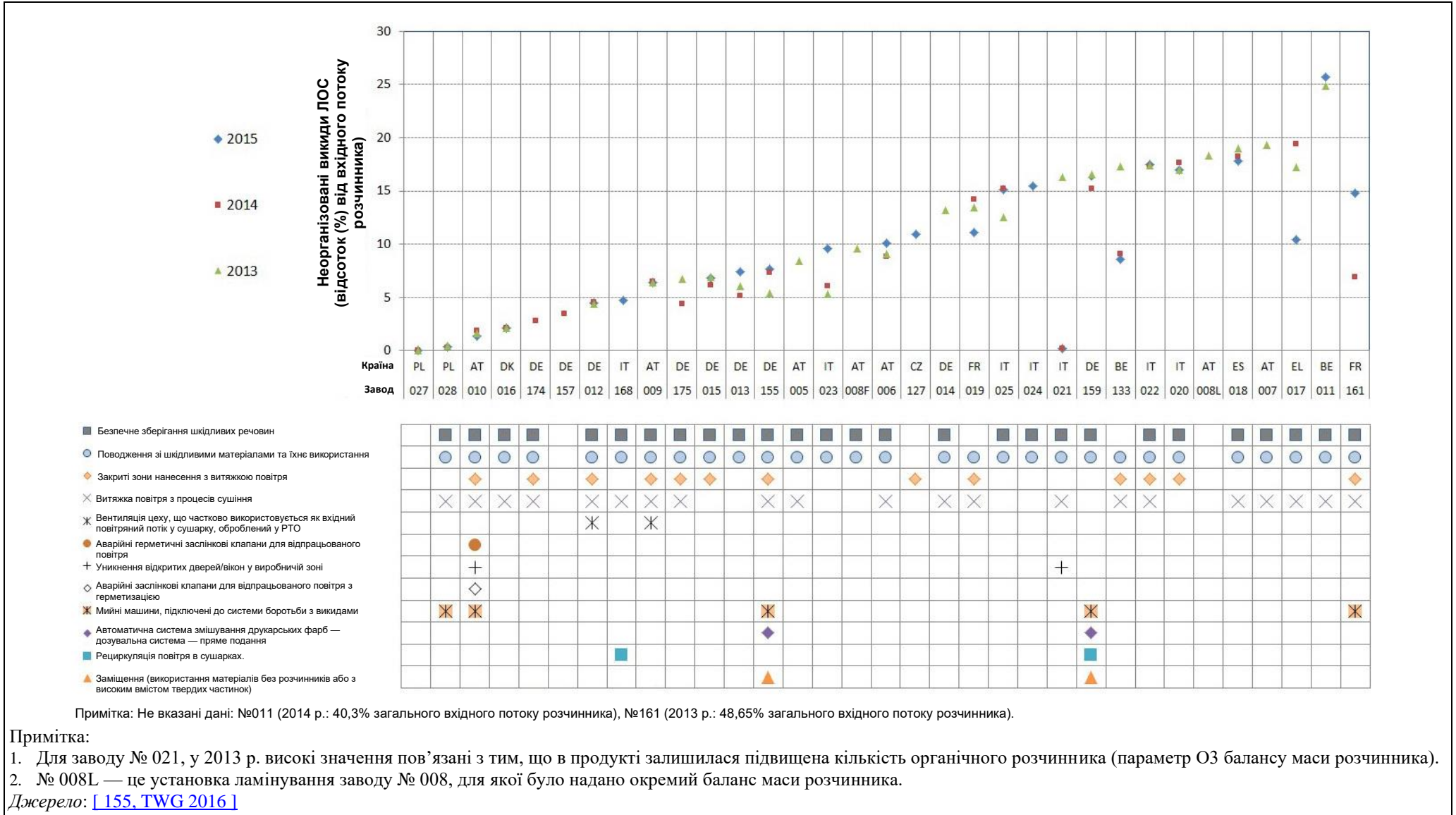
Рисунок 12.4: Неорганізовані викиди ЛОС, виражені як відсоток від вхідних потоків розчинника за період 2013–2015 рр.
