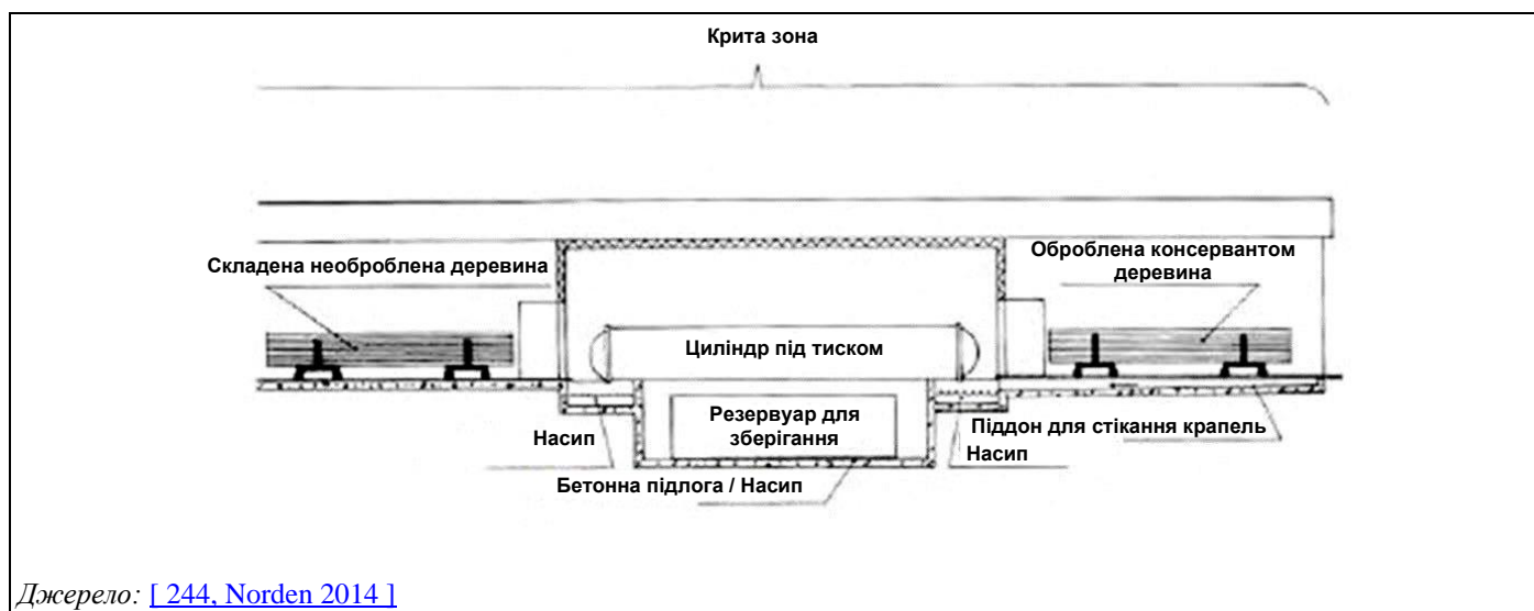
Рисунок 15.20: Схема, що демонструє різні варіанти запобіжних заходів (утримування, краплевловлювачі, покрівельні покриття)
