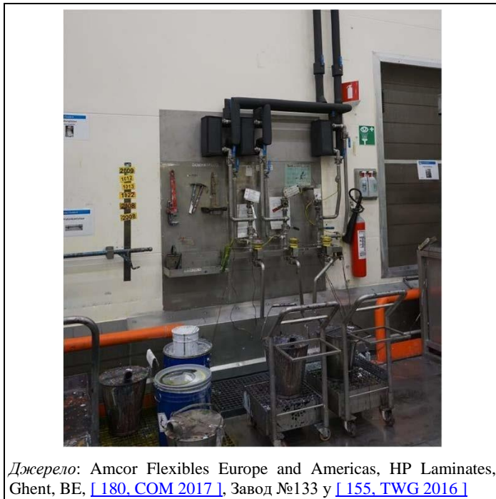
Рисунок 17.4: Автоматична система змішування на заводі флексографічного друку
