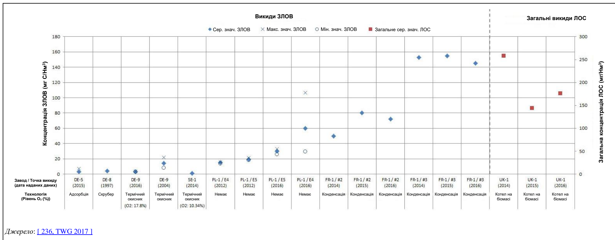
Рисунок 15.14: Повідомлені викиди ЛОС у відпрацьованих газах від заводів із використанням креозоту
