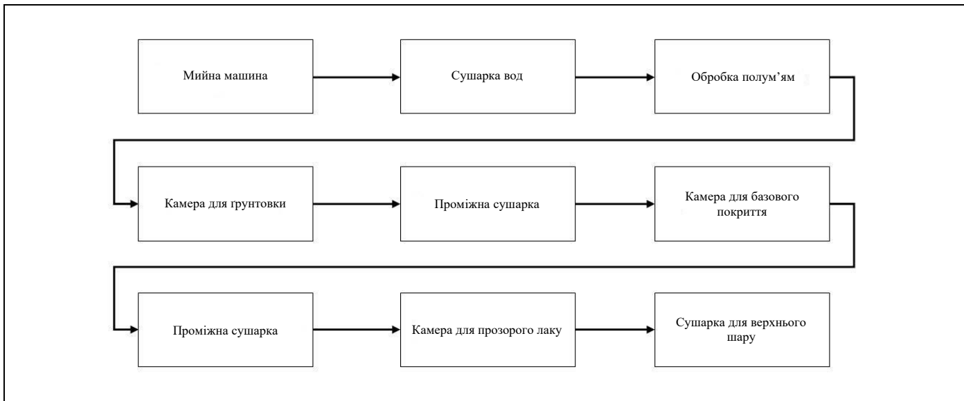
Рисунок 3.1: Процес нанесення покриття на водній основі на бампер
