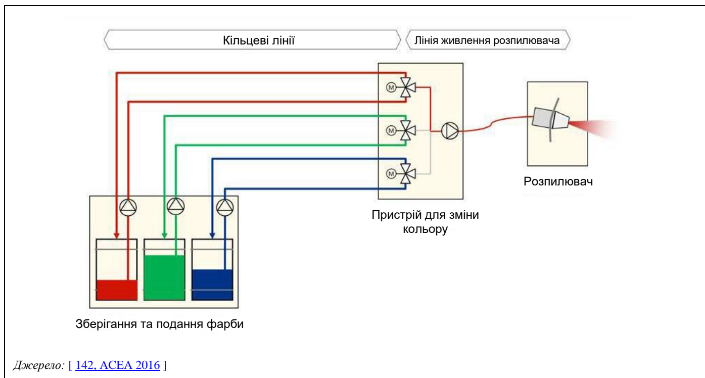
Рисунок 2.42: Схема різних частин системи подання фарби з кільцевими лініями
