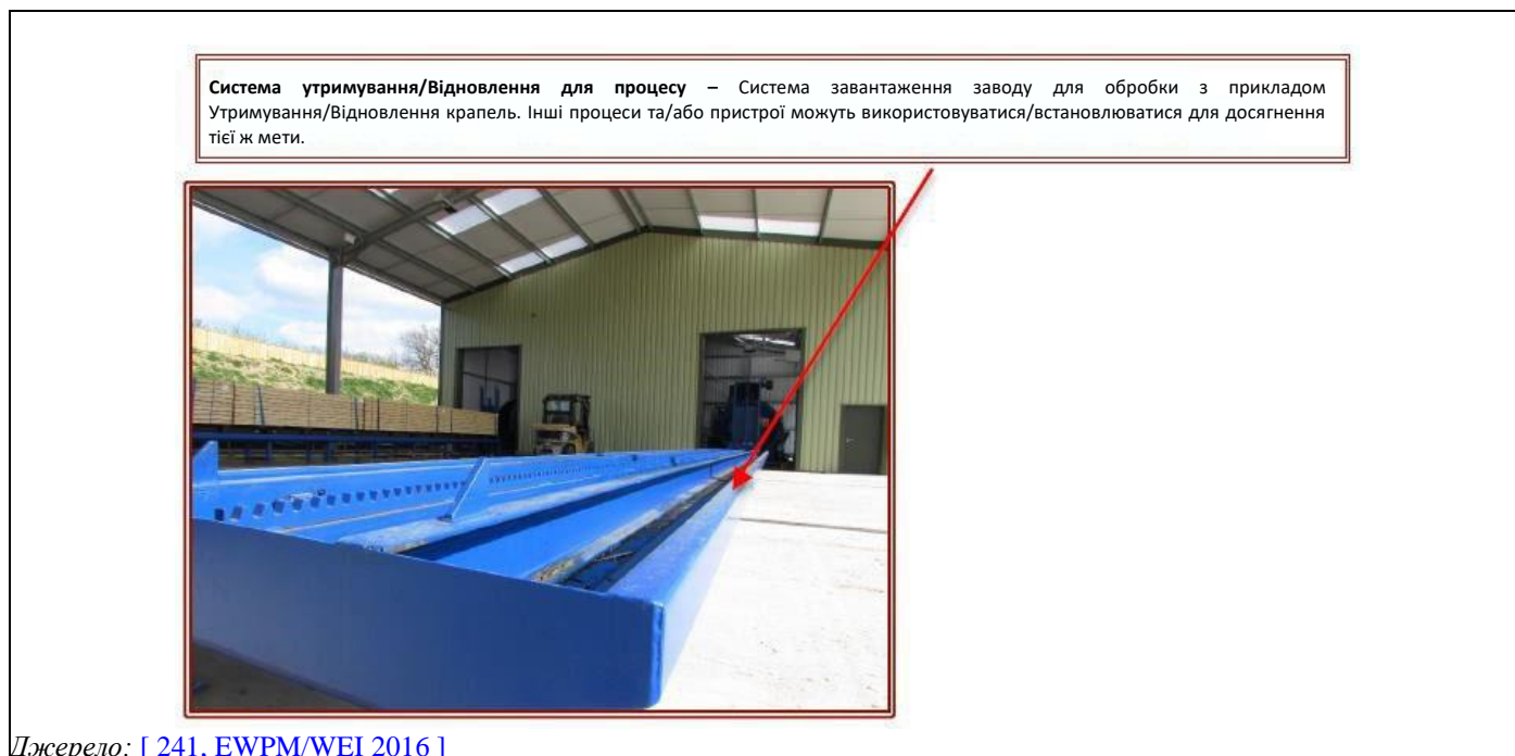
Рисунок 15.24: Приклад піддона, вбудованого в систему розвантаження (під зоною вилучення)
