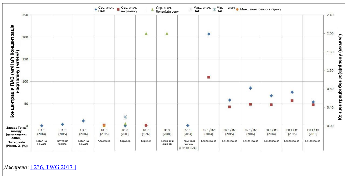
Рисунок 15.15: Повідомлені викиди ПАВ, нафталіну та бензо[а]пірену у відпрацьованих газах від заводів із використанням креозоту
