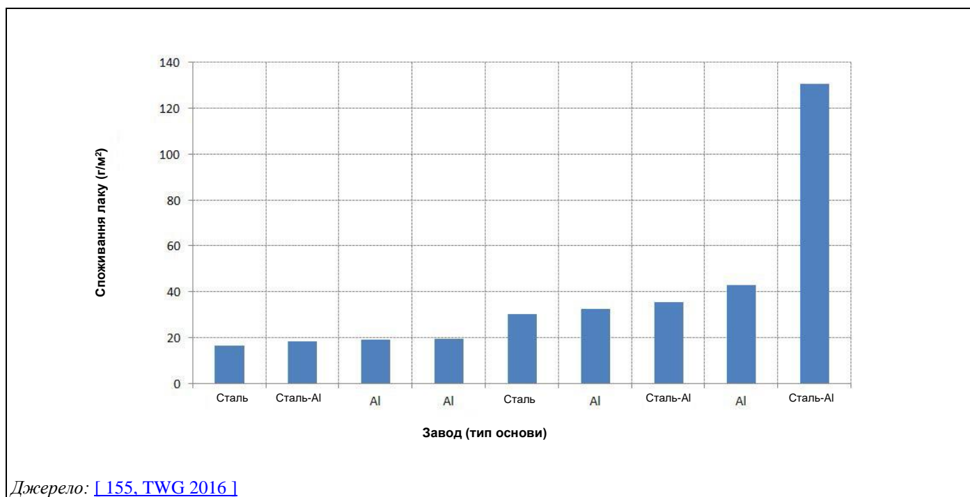
Рисунок 10.9: Споживання лаку установками для металевої упаковки (г споживання лаку на м 2 продукту) – Середні значення за період 2013–2015 рр.
