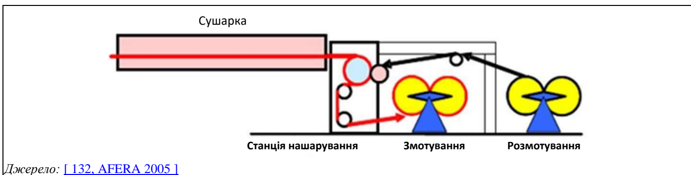
Рисунок 7.3: Установа нашарування
