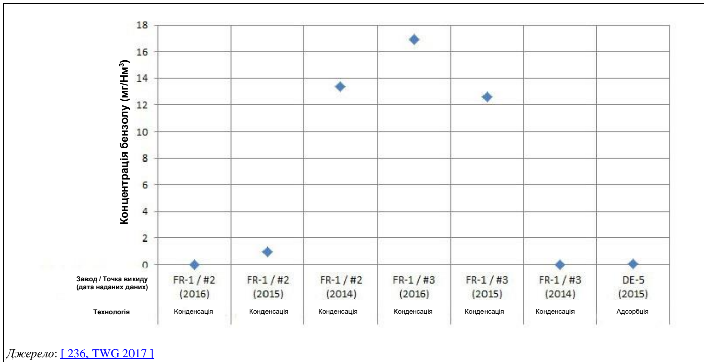
Рисунок 15.16: Повідомлені викиди бензолу у відпрацьованих газах від заводів із використанням креозоту
