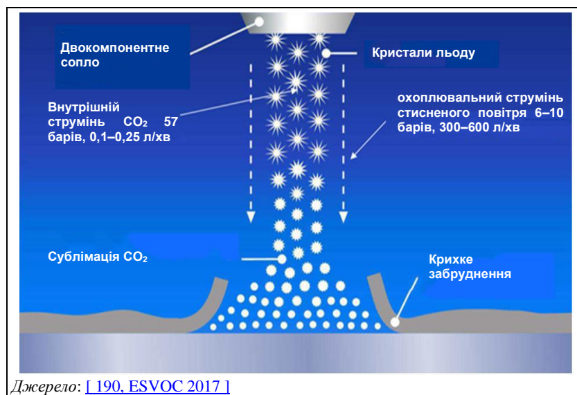
Рисунок 17.13: Викид рідкого CO 2
