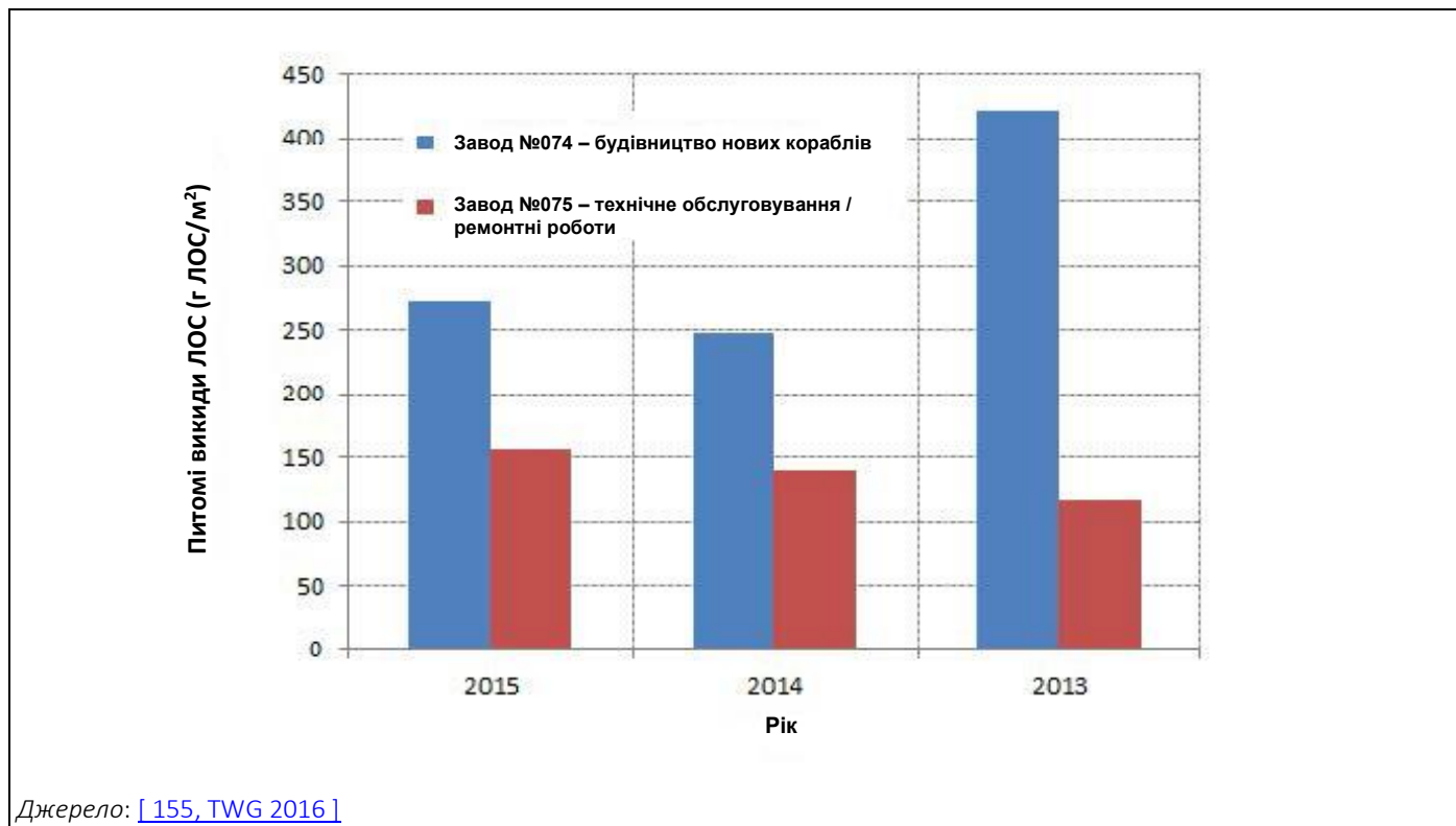
Рисунок 4.1: Загальні викиди ЛОС, виражені в г ЛОС на м 2 покритої поверхні для двох заводів за період 2013–2015 рр.
