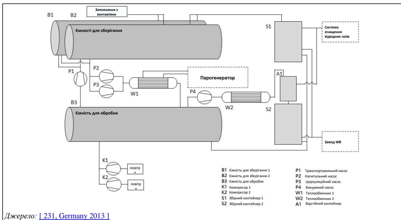
Рисунок 15.30: Схема заводу DE-1
