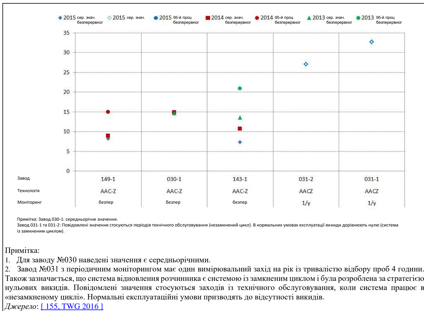
Рисунок 13.7: Викиди ЗЛОВ у відпрацьованих газах установки відновлення толуолу за період 2013–2015 рр.
