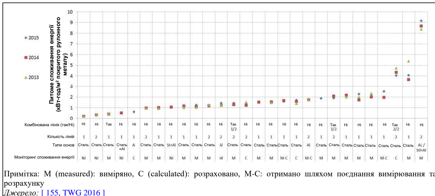
Рисунок 6.4: Питоме споживання енергії, виражене у кВт-год на м 2 покритого рулонного металу за період 2013–2015 рр.
