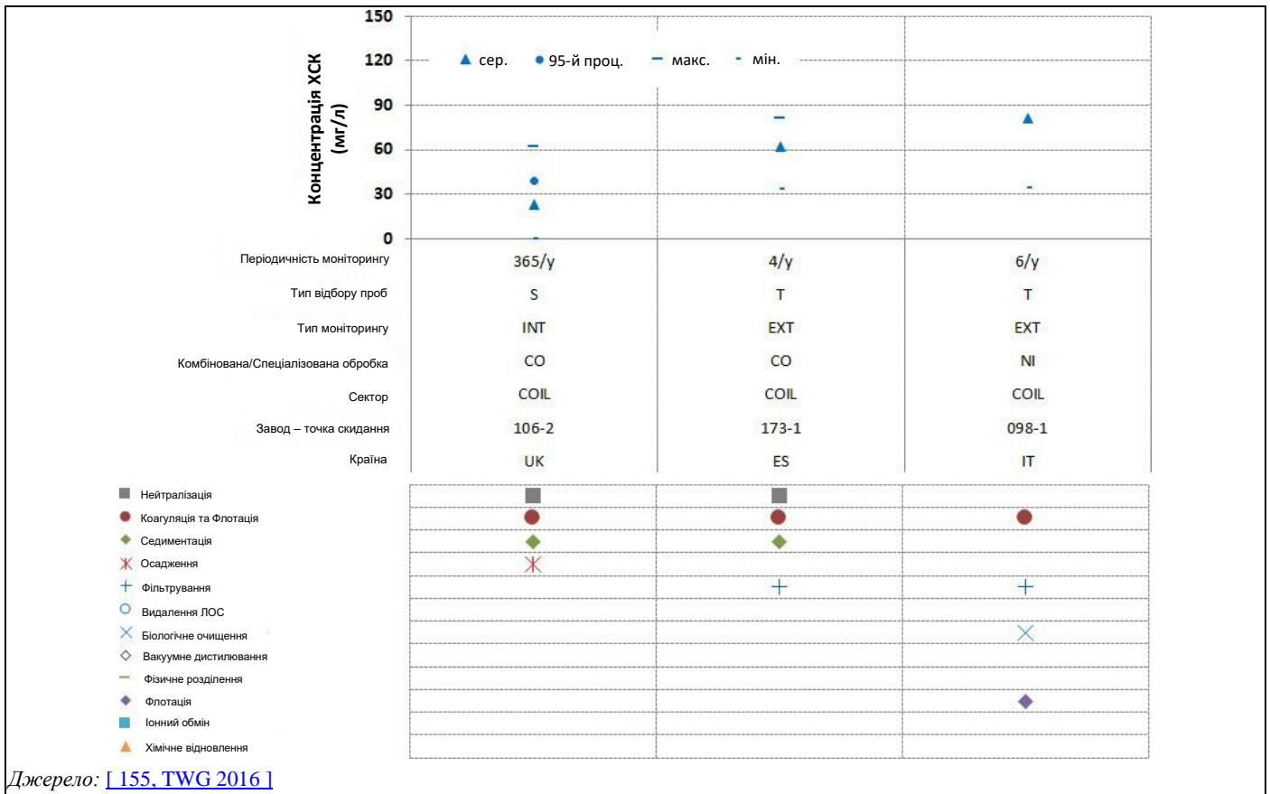
Рисунок 6.11: Значення концентрації ХСК для прямого скидання стічних вод заводів із нанесення покриття на рулонний метал (дані за 2015 р.)
