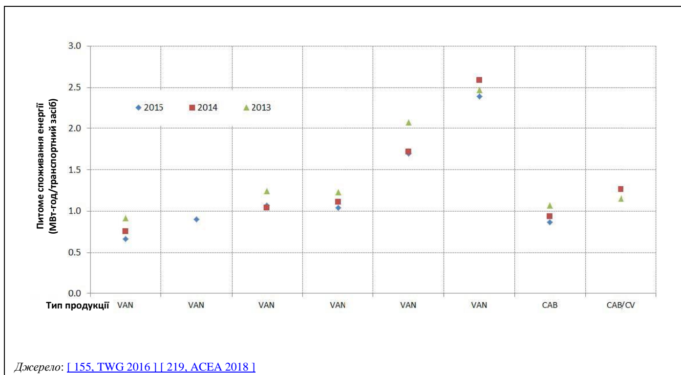
Рисунок 2.18: Питоме споживання енергії (МВт-год/транспортний засіб) для заводів із нанесення покриття на фургони, вантажні автомобілі та кабіни вантажного автомобіля
