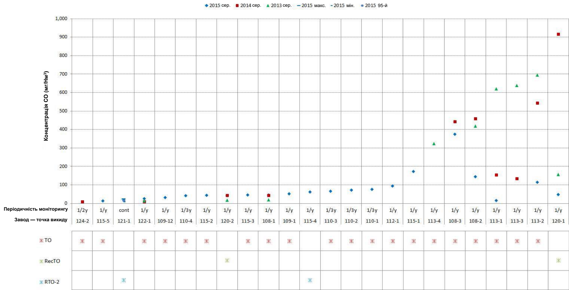
Рисунок 10.17: Викиди CO у відпрацьованих газах за період 2013–2015 рр.
