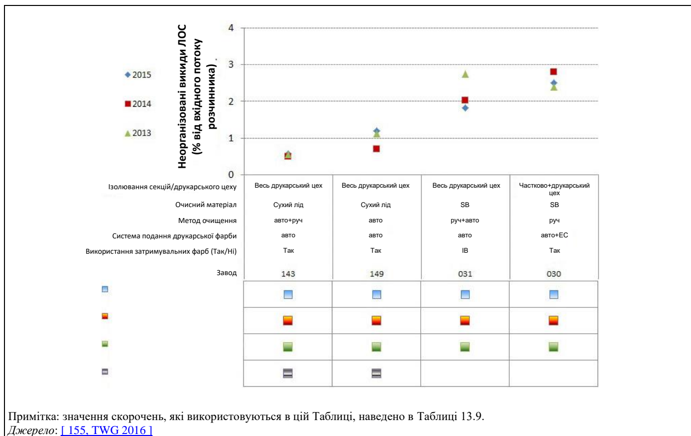
Рисунок 13.6: Неорганізовані викиди ЛОС, виражені як відсоток від вхідних потоків розчинника за період 2013–2015 рр.
