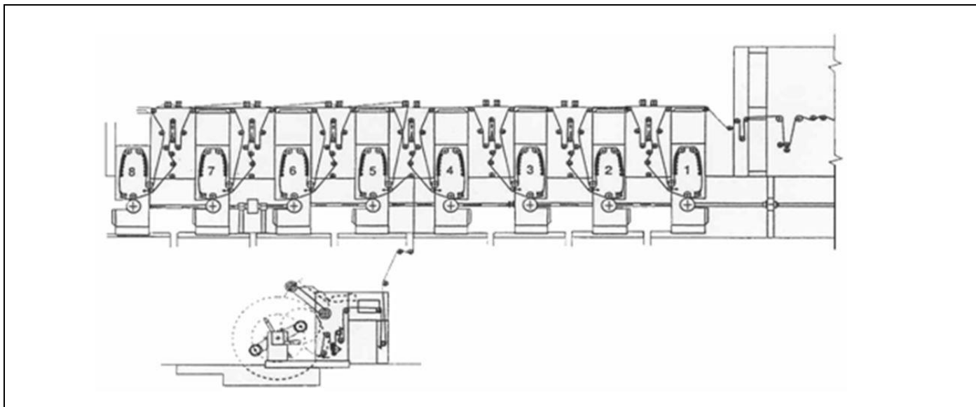
Рисунок 13.1: 4 + 4-колірна друкарська машина публікаційного ротогравюрного друку
