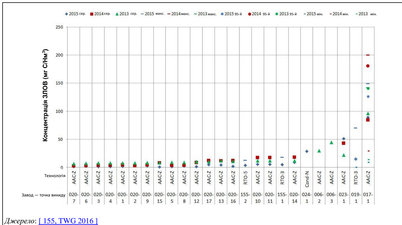
Рисунок 12.7: Викиди ЗЛОВ у відпрацьованих газах (безперервний моніторинг) за період 2013–2015 рр.
